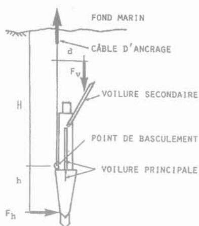
FIG. 1 Description et caractéristiques géométriques du système d'ancrage à forte capacité de tenue testé. Description and geometrical characteristics of the tested high holding capacity anchoring system.
