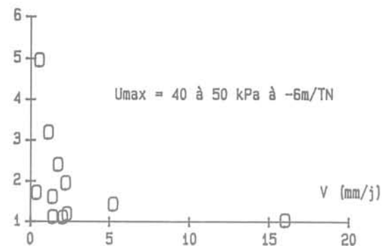
Fig. 8. — Relation U_{max}/U_0 en fonction de la vitesse maximum de déplacement.
