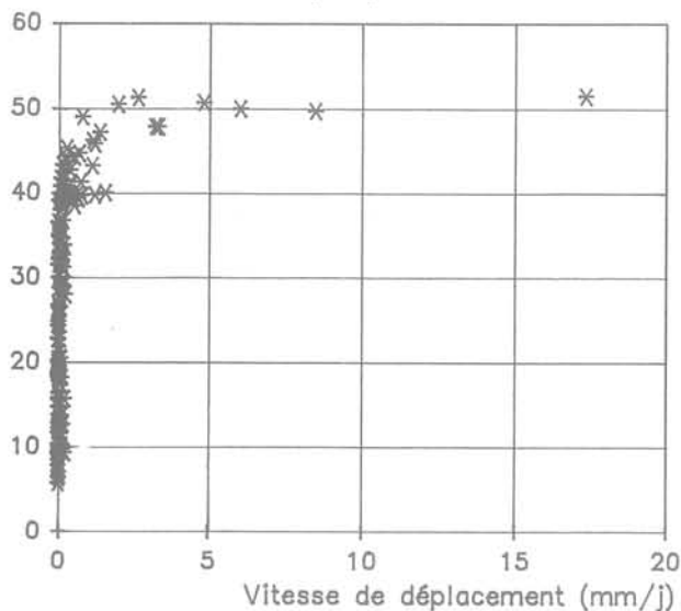
Fig. 6. — Relation pression interstitielle-vitesse de déplacement.
