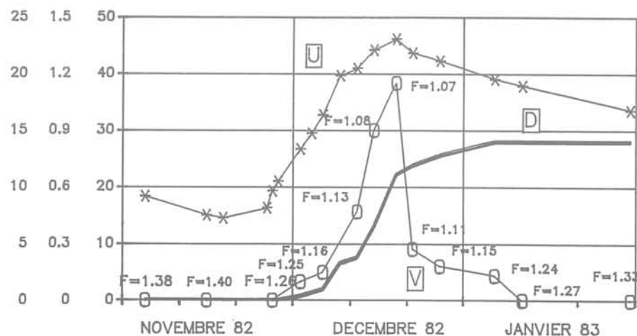
Fig. 7. — Evolution de la pression interstitielle, des déplacements et des vitesses de déplacement.
