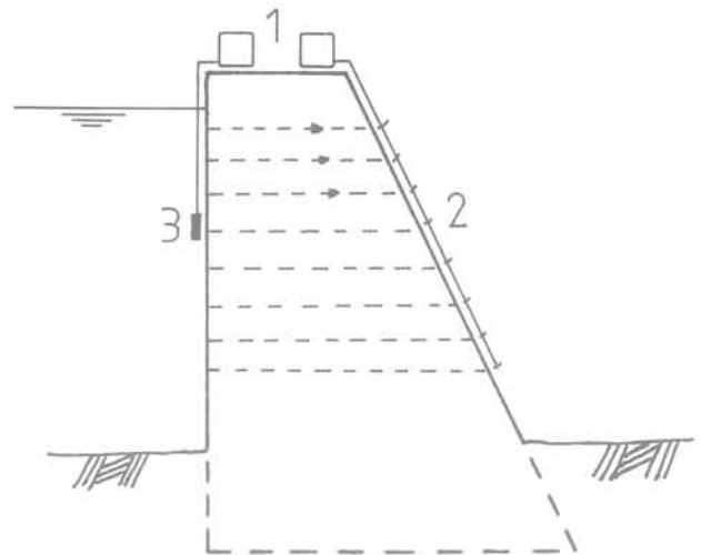
Fig. 5. — La transparence sismique.
