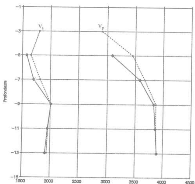
Fig. 10. et 11. — Barrage de la Gimond. Vitesses sismiques des ondes P et des ondes S.
