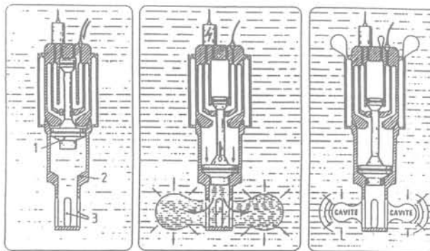
Fig. 1. — Principe de fonctionnement du canon à air.
