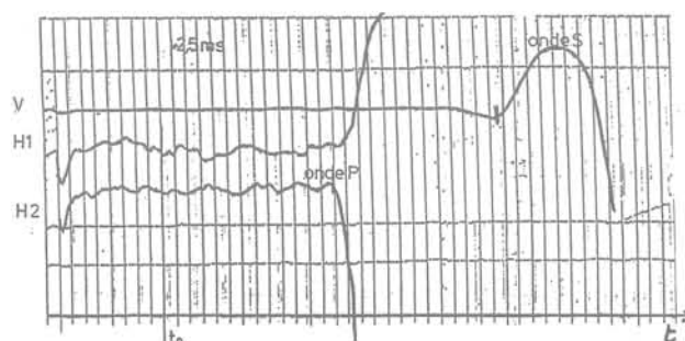
Fig. 8. — Exemple d'enregistrement fourni par une sonde composée de 3 géophones (1 V et 2 H). Barrage de la Gimond, S2-S1, 9 m de profondeur.
