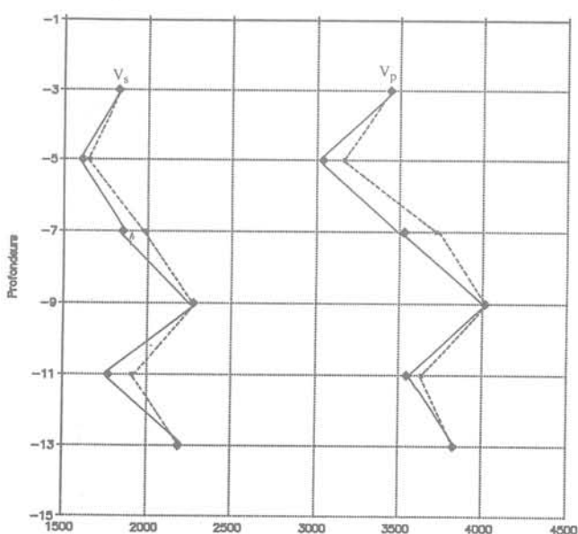
Fig. 10. et 11. — Barrage de la Gimond. Vitesses sismiques des ondes P et des ondes S.
