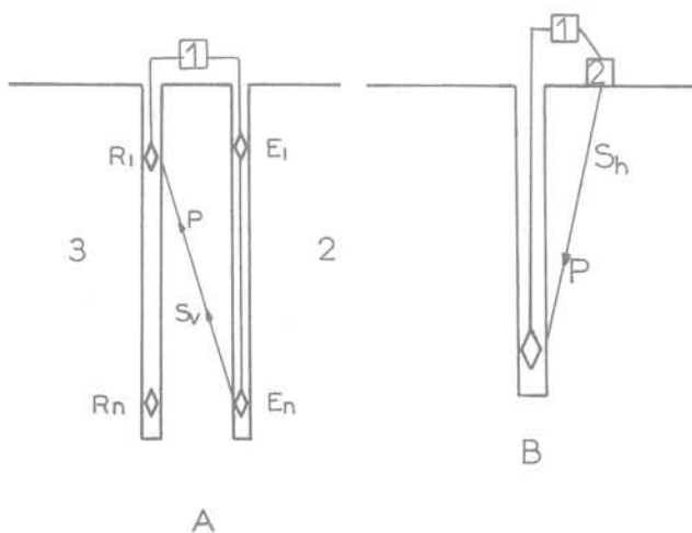
Fig. 4. — L'essai down-hole.
