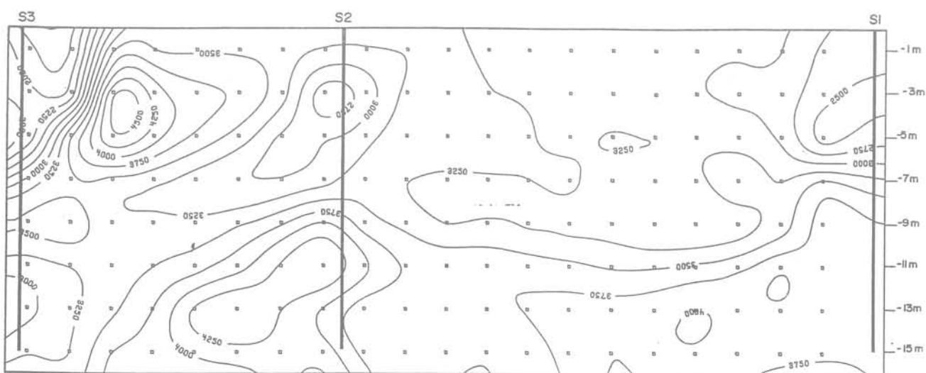
Fig. 9. — Barrage de la Gimond : carte des vitesses des ondes P, obtenue par tomographie.
