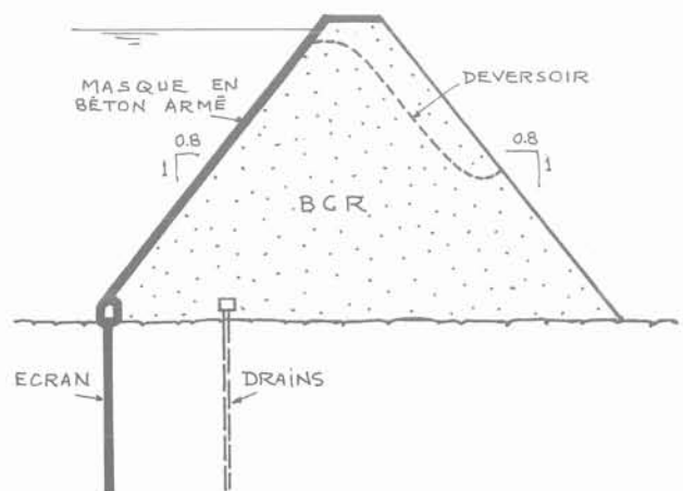
Fig. 1. — Barrage en BCR à profil symétrique.
