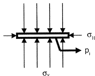
Distribution "réelle" des contraintes autour d'une armature à section rectangulaire
