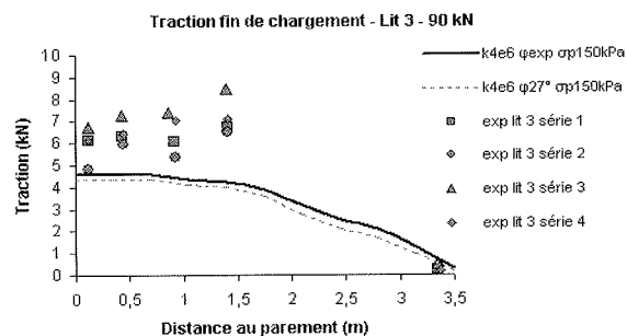
FIG. 7 Influence du frottement d'interface sur les efforts de traction des lits 1 et 3. Interface friction influence on tensile forces at the strip levels 1 and 3.
