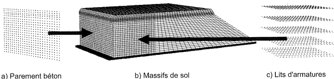
FIG. 1 Modèle numérique de l'ouvrage en Terre Armée : couches de sol (b) renforcées par les éléments du parement (a) et les lits d'armatures (c). Earth reinforced numerical model : soil layers (b) reinforced by concrete panels (a) and steel strips (c).
