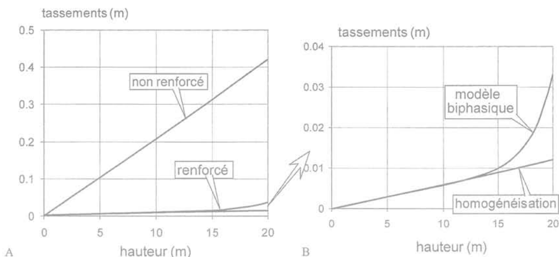
FIG. 12 Profils de tassement dans la couche de sol sur l'axe de symétrie. Settlement profiles along the symmetry axis.
