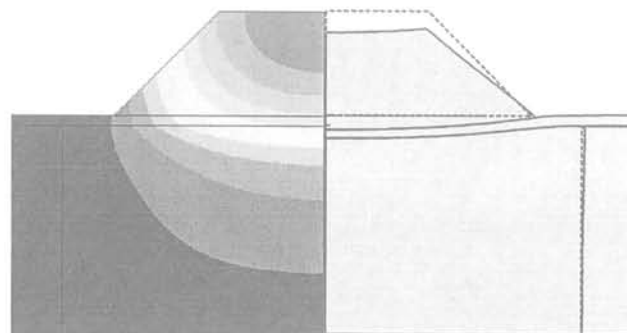
FIG. 11 Déformée de l'ouvrage et isovaleurs du tassement. Deformed configuration and contours of settlements.
