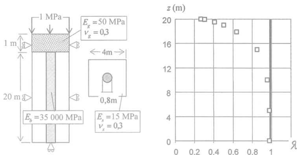
FIG. 3 Comparaison des facteurs de report de charge calculés respectivement par la méthode d'homogénéisation et la méthode des éléments finis (Rospars et al. , 2005).
