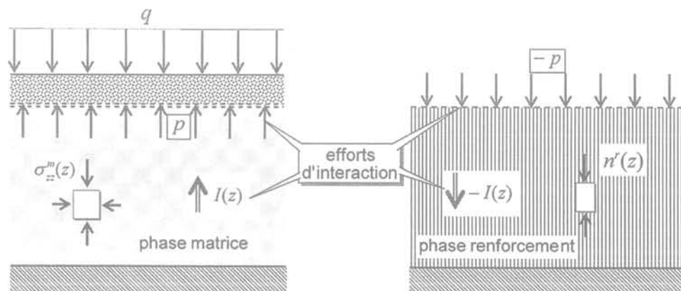
FIG. 5 Efforts intérieurs et extérieurs à chacune des phases. Stresses and external loads for each phase.
