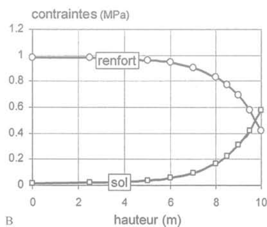
FIG. 9 Calage des courbes analytiques (traits pleins) et numériques (points). Fitting of analytical (solid lines) and numerical (points) curves.
