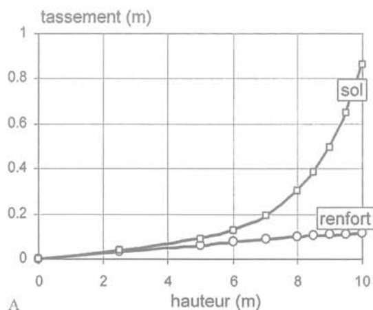
FIG. 9 Calage des courbes analytiques (traits pleins) et numériques (points). Fitting of analytical (solid lines) and numerical (points) curves.
