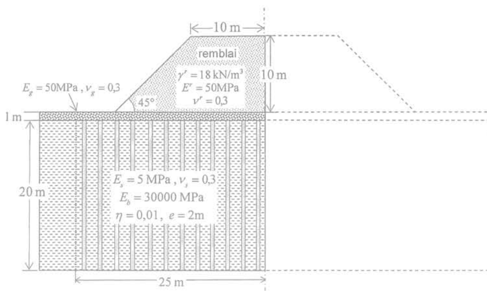
FIG. 10 Calcul du tassement d'un sol renforcé par inclusions rigides soumis à l'action du poids d'un remblai. Settlement analysis of a reinforced soil layer subject to the weight of an embankment.
