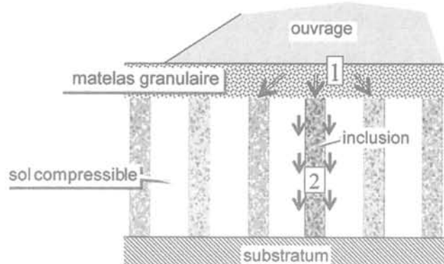
FIG. 1 Schéma de principe de la technique de renforcement d'un sol de fondation par inclusions rigides.
