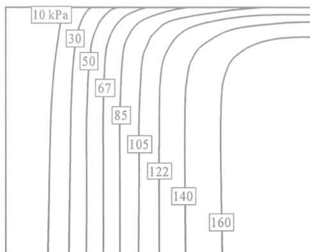
FIG. 13 Isovaleurs de la contrainte de compression dans la phase renforcement. Contours of compressive stress in the reinforcements.
