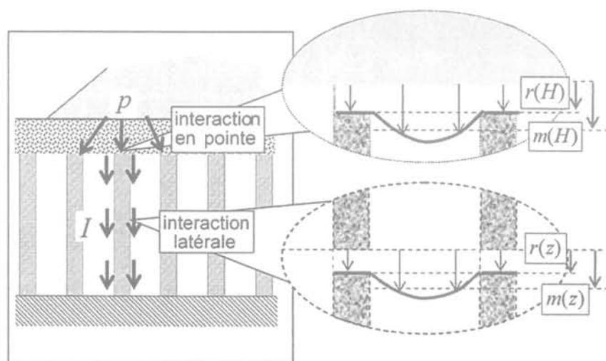
FIG. 7 Principe de l'identification des coefficients d'interaction du modèle biphasique. Identification of interaction coefficients for the two-phase model.
