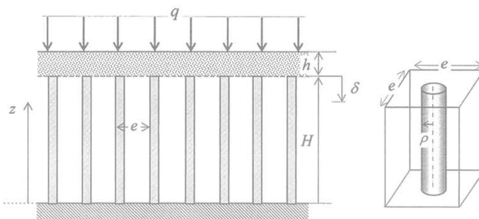
FIG. 2 Analyse du tassement sous charge uniforme d'une couche de sol renforcée par une distribution régulière d'inclusions rigides. Settlement analysis of a reinforced soil layer under uniform surface loading.
