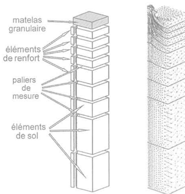
FIG. 8 Maillage par éléments finis du quart de la cellule élémentaire de sol renforcé (Cartiaux, 2006). Finite element mesh of the reinforced soil elementary cell.
