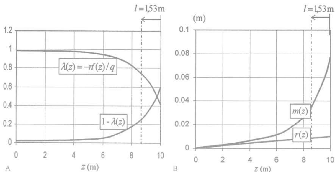
FIG. 6 Profils de tassements et de contraintes dans les phases matrice et renforcement. Settlement profiles and stress distributions in the matrix and reinforcement phases.
