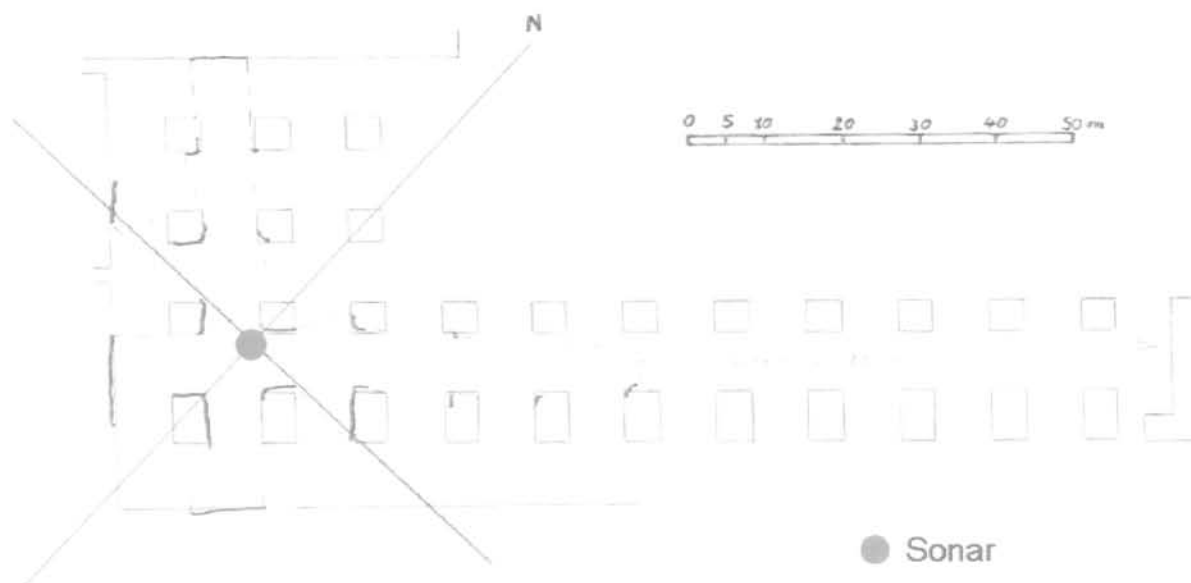
FIG. 12 Plan de la mine de Dieuze et résultats du relevé sonar. Dieuze mine map and sonar survey measurements.
