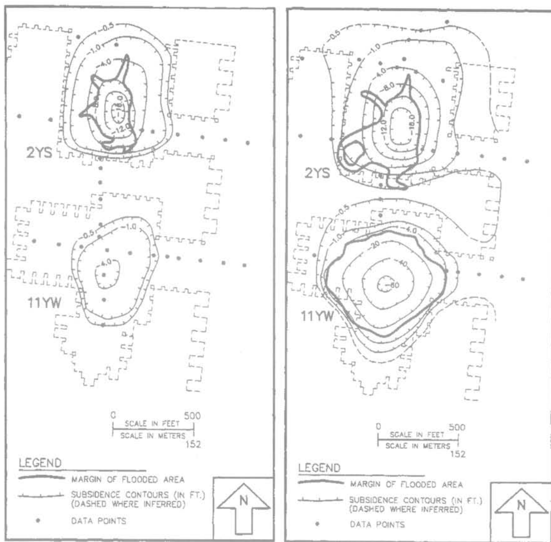
FIG. 5 Subsidence de surface les 14 avril 1994 (gauche) et 13 au 13 juin 1995 (droite) au-dessus des quartiers 2YS et 11YW de la mine de Retsof. Les chambres ont une hauteur de 12 pieds (3,6 m) ; la cuvette au-dessus du quartier 11 YW finira par atteindre 70 pieds (21 m) de profondeur (d'après Gowan et Trader, 2000). Surface subsidence as of April 14, 1994 (left) and as of June 13 and 15, 1994 (right) above the 2YS and 11YW panels of the Retsof mine. Rooms are 12 feet high. The final sinkhole depth above the 11 YW panel will be 70 feet (after Gowan and Trader, 2000).
