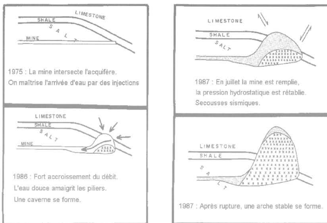
FIG. 9 Scénario possible des événements à la Potash Company of America Mine, Saskatoon (d'après Gendzwil et Prugger, 1990). Proposed sequence of events for Potash Company of America Mine, Saskatoon (After Gendzwil and Prugger, 1990).
