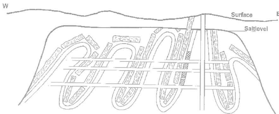
FIG. 4 Coupe du dôme de sel de Ronnendorf (d'après Rölleke, 2000). Vertical cross-section of the Ronnendorf salt dome (After Rölleke, 2000).
