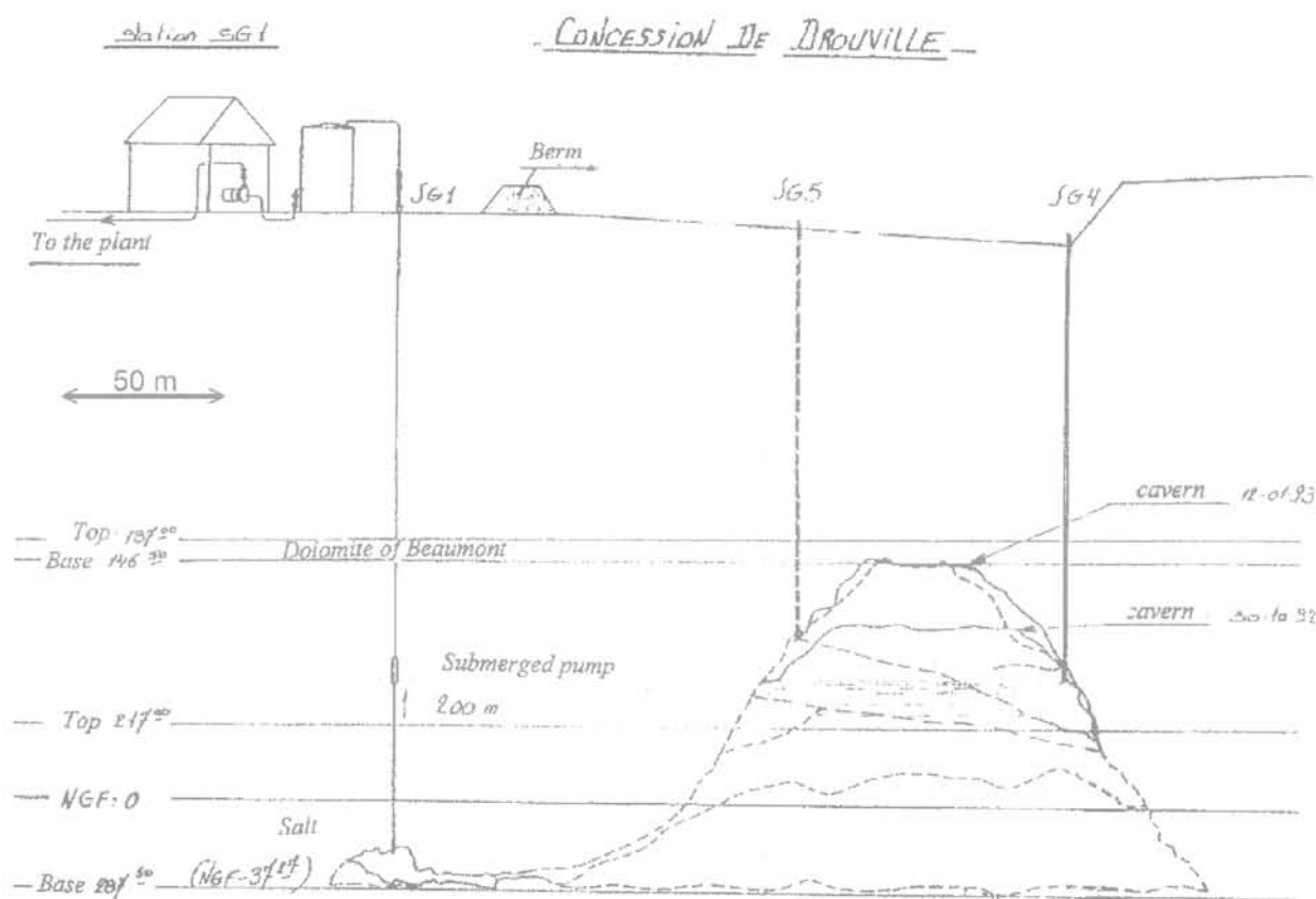
FIG. 7 Pompage de la saumure dans les cavernes SG4-SG5 (concession de Drouville). Le toit de la caverne remonte jusqu'à la Dolomie de Beaumont, atteinte en 1992. On décide alors de décompresser la caverne en descendant le niveau de saumure dans le puits SG1 au moyen d'une pompe immergée. La chute de pression dans la caverne n'a pas provoqué l'effondrement (d'après Buffet, 1998). Brine withdrawal from the SG4-SG5 caverns (Drouville concession). Cavern roof rises through stoping and reaches the Beaumont Dolomite by 1992. It was decided to lower brine level in SG1 well. A submerged pump was used. Pressure drop did not provoke cavern failure (After Buffet, 1998).
