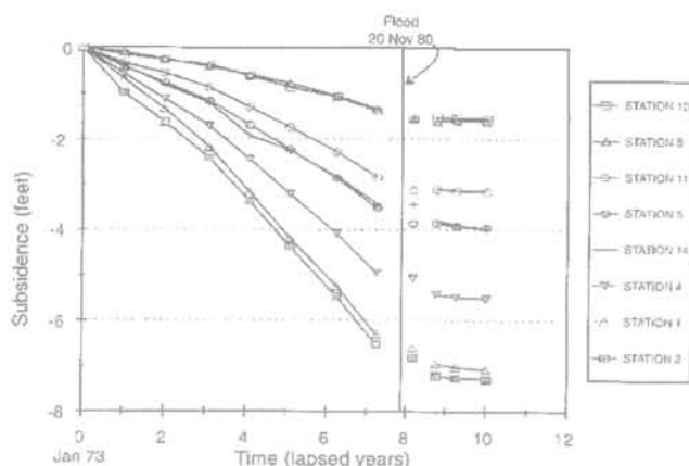
FIG. 8 Subsidence avant et après l'ennoyage de la mine de Jefferson Island (d'après Van Sambeek et Thoms, 2000). Pre-and post-flooding surface subsidence at Jefferson Island salt mine (After Van Sambeek and Thoms, 2000).
