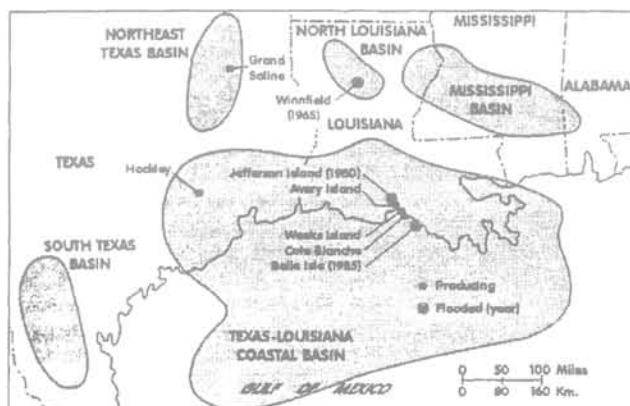
FIG. 1 Mines et dômes de sel au Texas et en Louisiane. L'année indiquée est celle de la perte de la mine (d'après Johnson et Gonzales, 1978, cité par Thoms et Gehle, 2000). Salt mines and salt domes in Louisiana and Texas (After Johnson and Gonzales, referred by Thoms and Gehle, 2000).
