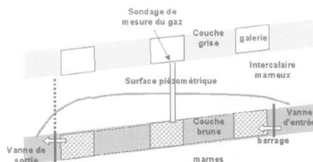
FIG. 6 Coupe schématique du dispositif de surveillance de l'atmosphère au cours de l'ennoyage du site pilote de Tressange.
