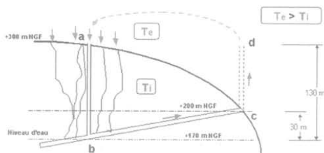
FIG. 4 Schéma de principe du tirage naturel en période estivale (contexte du réservoir de Moyeuve-Grande).
