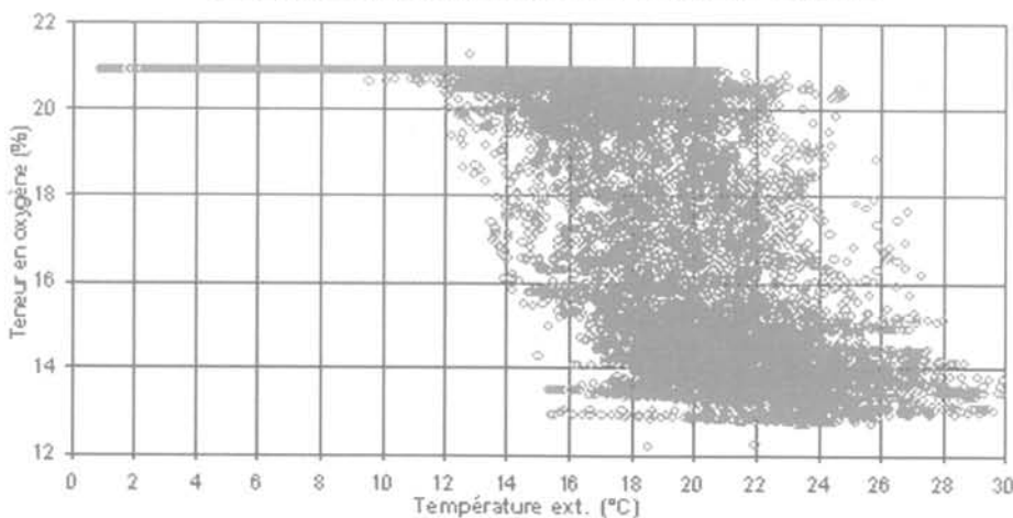
FIG. 5 Corrélation entre la température extérieure et les teneurs en O_2 et CO_2 observées dans un orifice du réservoir de Moyeuve-Grande.
