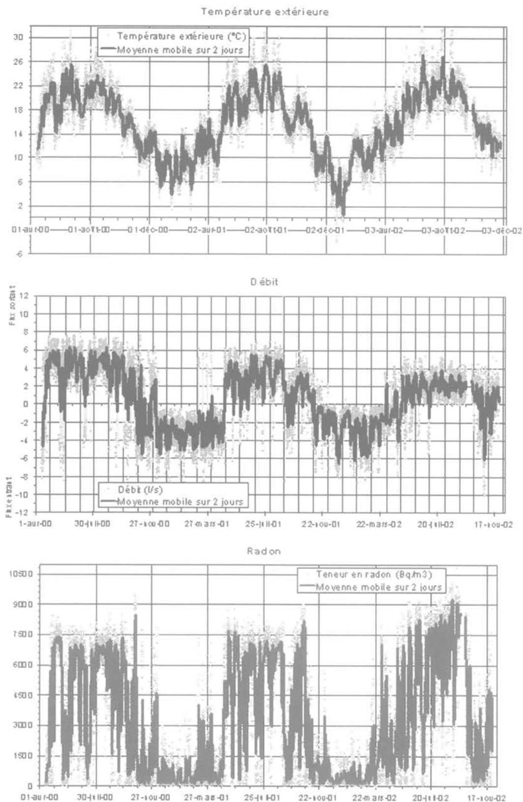
FIG. 2 Évolution de la température extérieure, du débit d'air et de la teneur en radon observés dans une galerie débouchant du réservoir de Moyeuivre-Grande. Outside temperature, air flow rate and radon content evolutions observed in a gallery connected to the Moyeuivre-Grande reservoir.
