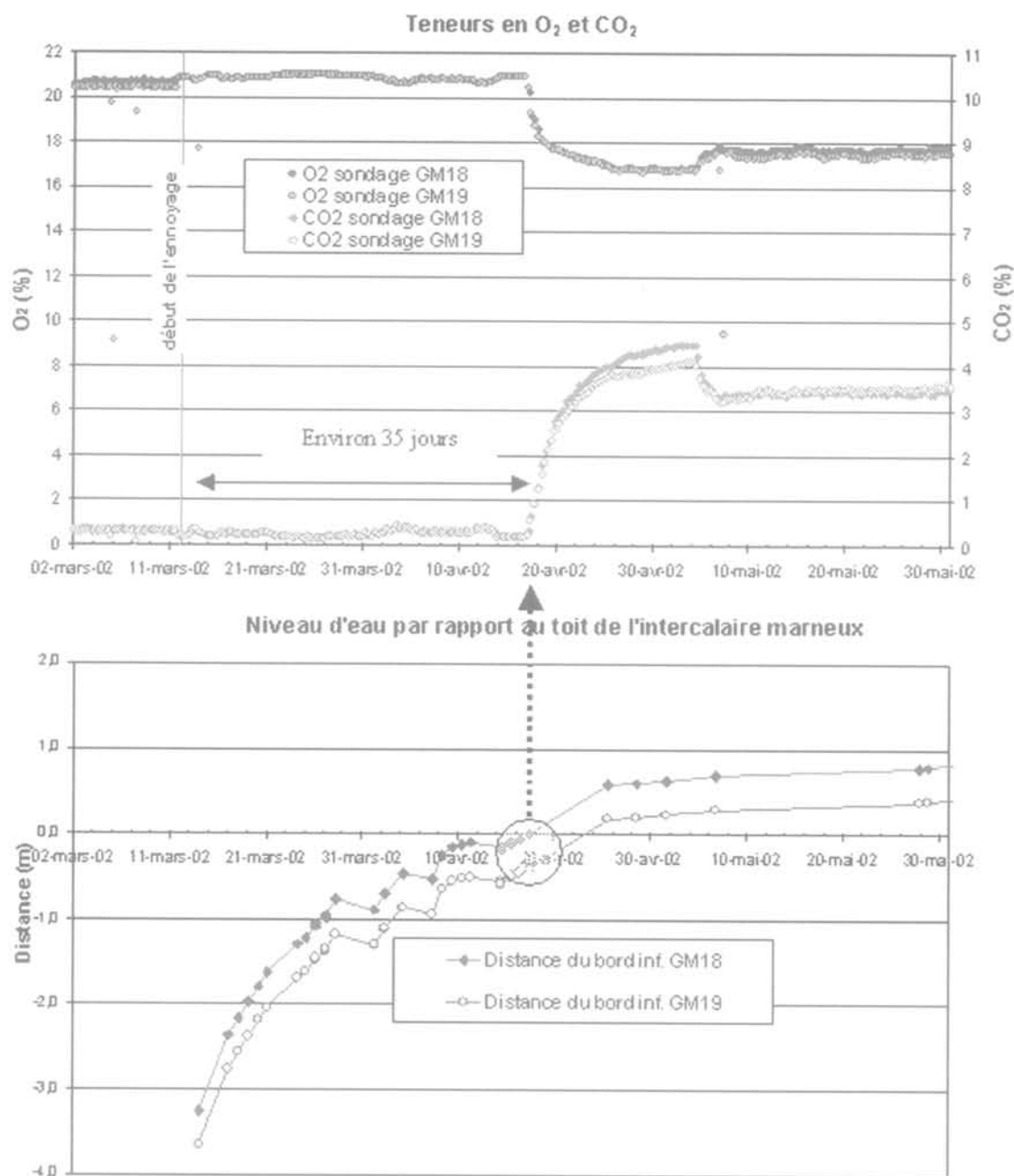
FIG. 7 Évolution de la composition gazeuse dans le massif, au cours de l'ennoyage du site pilote de Tressange.
