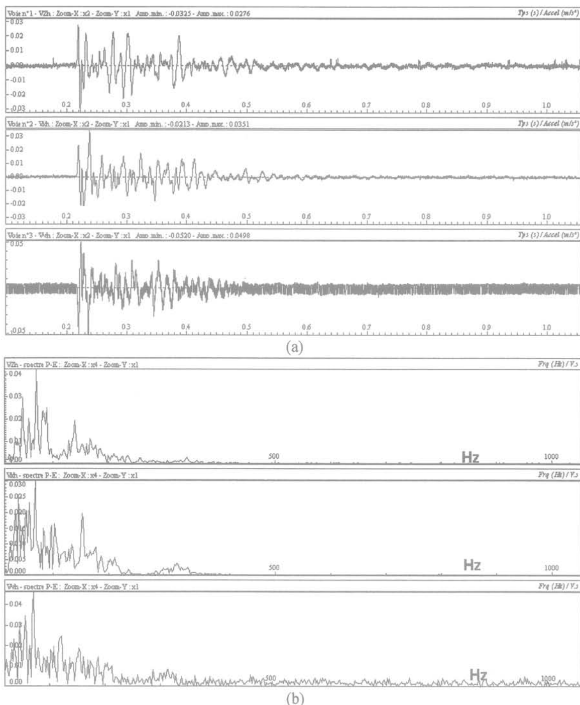
FIG. 5 Exemple de signal microsismique caractéristique d'un tir d'explosif: (a) signal temporel en accélération ( m/s^2 ) sur trois axes X, Y, Z; (b) contenu spectral (Senfaute et al. , 2000). Example of seismic signal recorded during blasting operations: (a) seismogram according to X, Y, Z of accelerations ( m/s^2 ) and (b) frequency spectra (Senfaute et al. , 2000).
