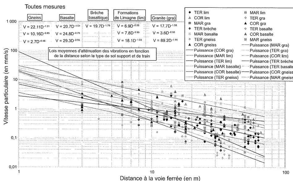
FIG. 1 Vitesse particulaire mesurée en 2006 sur 29 sites de la région Auvergne au passage de 133 trains différents (source CETE Lyon). Particle velocity measured in 2006 for 29 sites at the passage of 133 different trains in the Auvergne region (source CETE Lyon).
