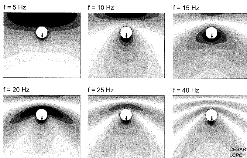
FIG. 7 Vibrations induites autour d'un tunnel par le passage d'un train : modélisation par la méthode des éléments de frontière (Semblat et Dangla, 2005).
