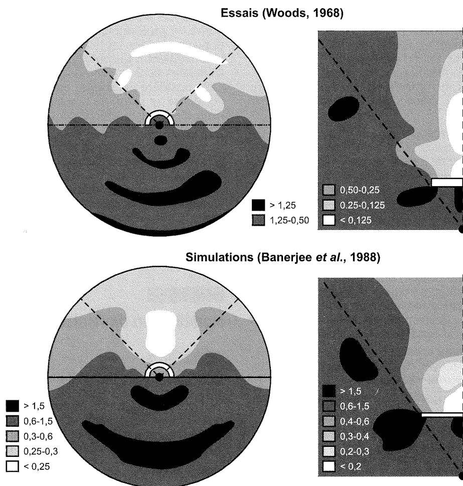
FIG. 9 Isolation vibratoire à l'aide d'une tranchée circulaire (gauche) ou rectiligne (droite) : résultats expérimentaux de Woods (1968) et numériques de Banerjee et al. (1988), d'après Semblat et Pecker (2009). Vibration isolation using a circular (left) or linear (right) trench : experimental results from Woods (1968) and numerical ones from Banerjee et al. (1988), from Semblat & Pecker (2009).
