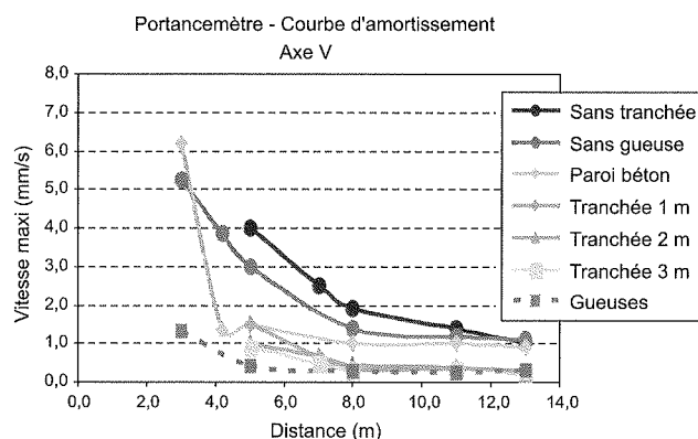
FIG. 11 Comparaison des différents dispositifs atténuant les vibrations pour le portancemètre et la composante verticale. Comparison of various isolation systems for the vertical component (portancemeter loading).
