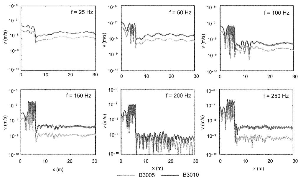
FIG. 13 Résultats des simulations par la méthode des éléments de frontière du LCPC pour les cas-tests d'isolation vibratoire RATP/CSTB (Grasso, 2008). Results of the BEM simulations performed at LCPC for the RATP/CSTB vibration isolation test-cases (Grasso, 2008).
