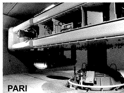
FIG. 3 Dispositif expérimental pour les essais sur modèles réduits en centrifugeuse : LCPC Nantes, université de Cambridge, centre C-Core à Terre-Neuve, PARI au Japon (Semblat et Pecker, 2009). Experimental facilities for reduced scale centrifuge experiments : LCPC Nantes, University of Cambridge, C-Core center in New Foundland, PARI in Japon (Semblat & Pecker, 2009).
