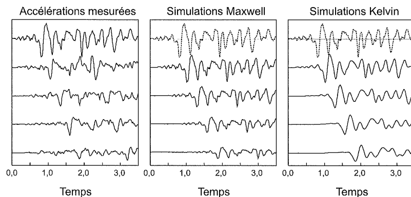
FIG. 4 Signaux d'accélération mesurés en centrifugeuse (gauche) et simulations viscoélastiques à l'aide d'un modèle de Maxwell (centre) et d'un modèle de Kelvin (droite), d'après (Semblat et Luong, 1998). Acceleration signals measured in the centrifuge (left) and viscoelastic simulations considering a Maxwell (center) and Kelvin (right) model (Semblat & Luong, 1998).
