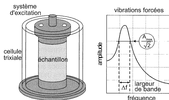
FIG. 2 Caractérisation dynamique des sols en laboratoire : dispositif de colonne résonnante (gauche) et réponse typique d'un échantillon en vibration forcée (droite). Dynamic characterization of soils in the lab : resonant column test (left) and typical specimen response in forced vibrations (right).
