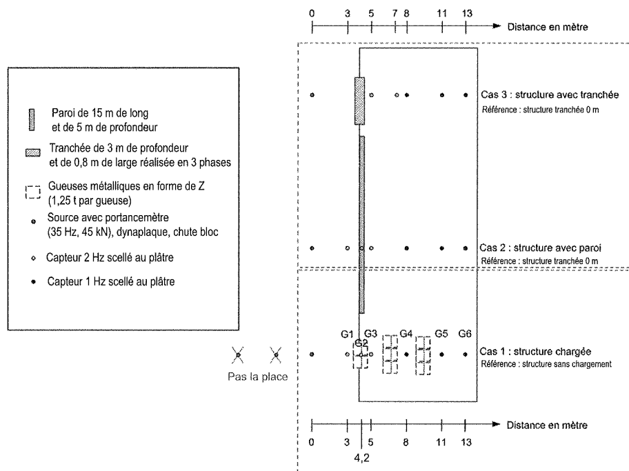
FIG. 10 Implantation du dispositif expérimental pour évaluer trois systèmes amortissants (Jacqueline, 2009).
