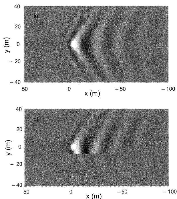
FIG. 14 Modélisation d'un système d'isolation par tranchée dans le cas de vibrations ferroviaires (Karlström et Boström, 2007) : pas d'isolation (en haut), une tranchée (en bas).
