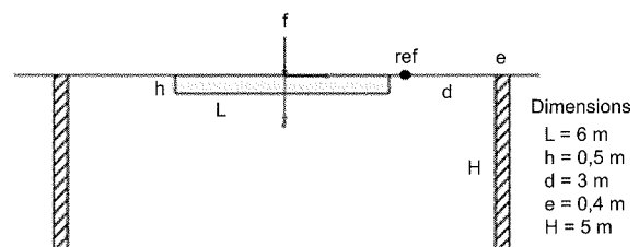
FIG. 12 Configuration géométrique typique des cas-tests d'isolation vibratoire proposés par la RATP et le CSTB (Coquel, 2008). Typical geometrical configuration to study vibration isolation as proposed by RATP and CSTB (Coquel, 2008).
