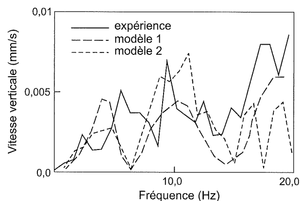
FIG. 8 Comparaison entre le calcul et l'expérience sur un tunnel réel (Semblat et Dangla, 2005).
