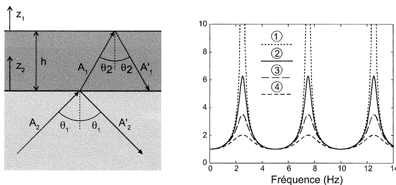
FIG. 5 Amplification d'une onde plane dans une couche de sol (Semblat et Pecker, 2009) : définition des différentes ondes (gauche) et fonction de transfert pour différents rapports de célérités (droite). Amplification of a plane wave in a soil layer (Semblat & Pecker, 2009) : definition of the various waves (left) and transfer function for different velocity ratios (right).
